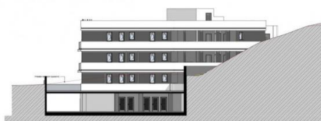
ELEVATION 4 SCALE: 1:100
